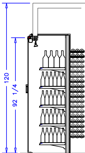
DOOR (A) SECTION
