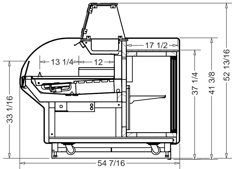
SECTION A-A SCALE 0.06 : 1
